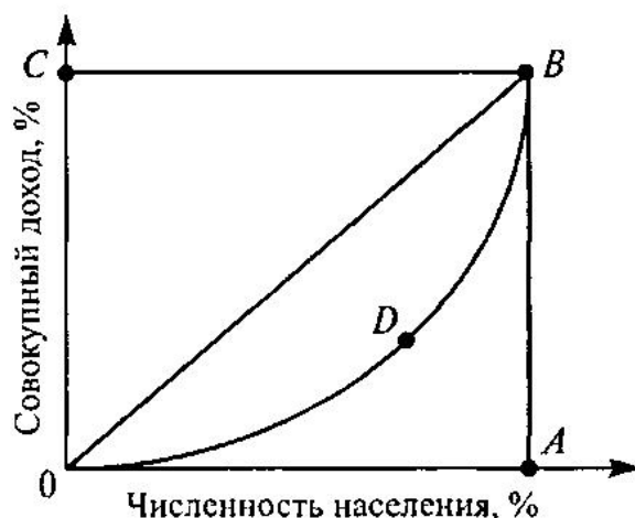
Рисунок 1 – Кривая Лоренца
